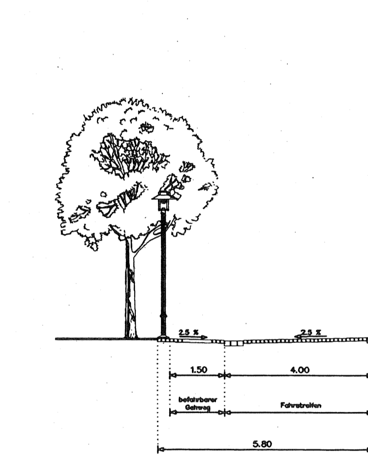
STRASSENPROFIL 1:100
